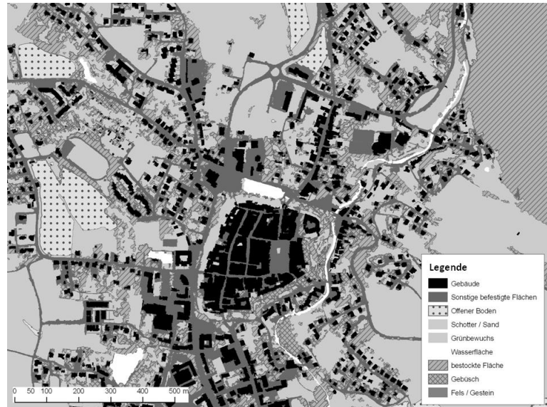
Abb.1: Ergebnis der Landbedeckungskartierung für den Raum Freistadt, Oberösterreich Aus Gründen der Übersichtlichkeit sind in der Legende nur die in diesem Ausschnitt vorkommenden Landbedeckungsklassen (9 von insgesamt 17) dargestellt.
